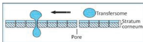
شکل ۳- نمایش نفوذپذیری ترانسفرزوم از طریق منافذ لایه شاخی پوست.
