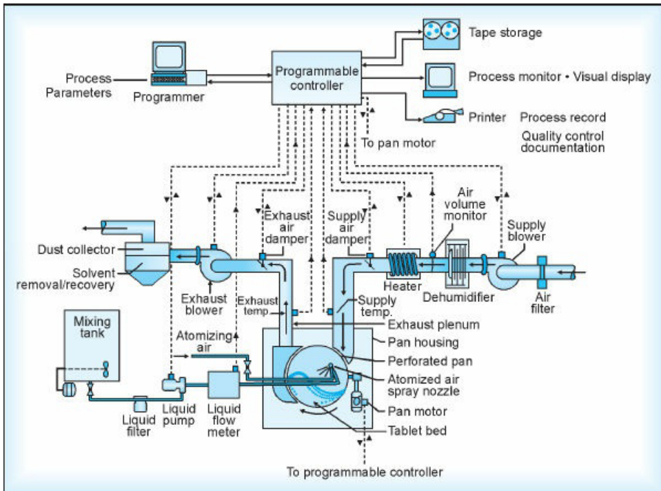
شکل ۵- نمایش نموداری سیستم روکش‌دهی خودکار.
