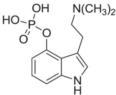
Psilocybin
