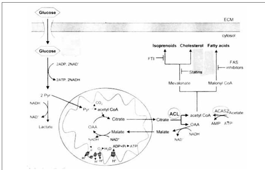
شکل ۳ - مهار ACL باعث مهار تولید استیل کوآنزیم A و مهار دوباره پر شدن (Replenishing) گز الواستیک اسید (OAA) در سیکل کرپس می‌شود.
